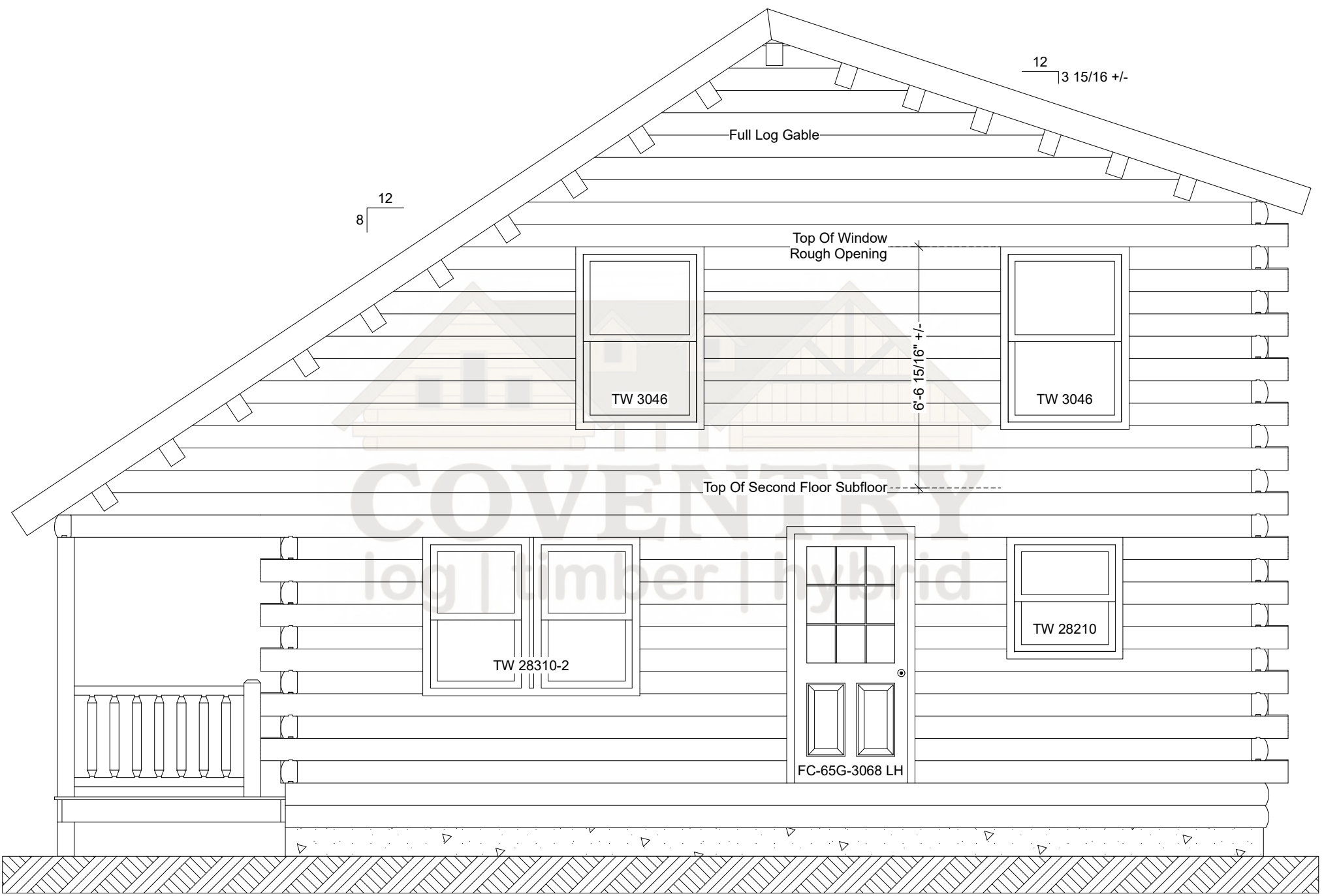
Andover Right Elevation
