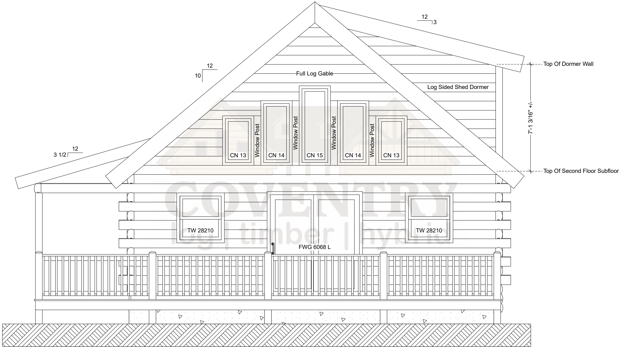
Ascutney Right Elevation
