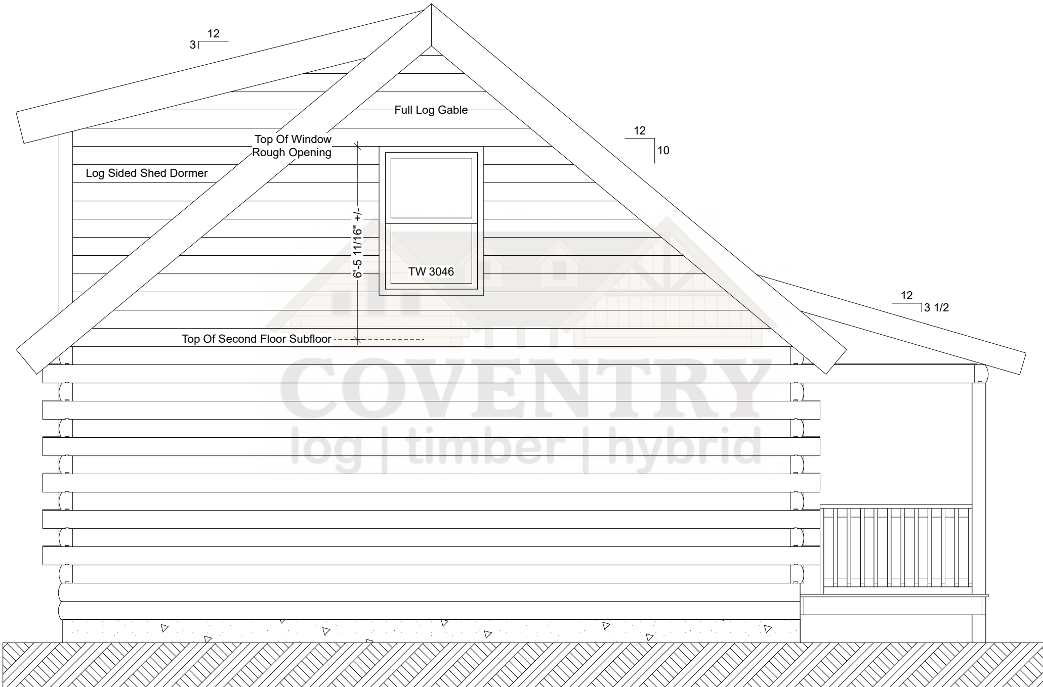
Ascutney Left Elevation
