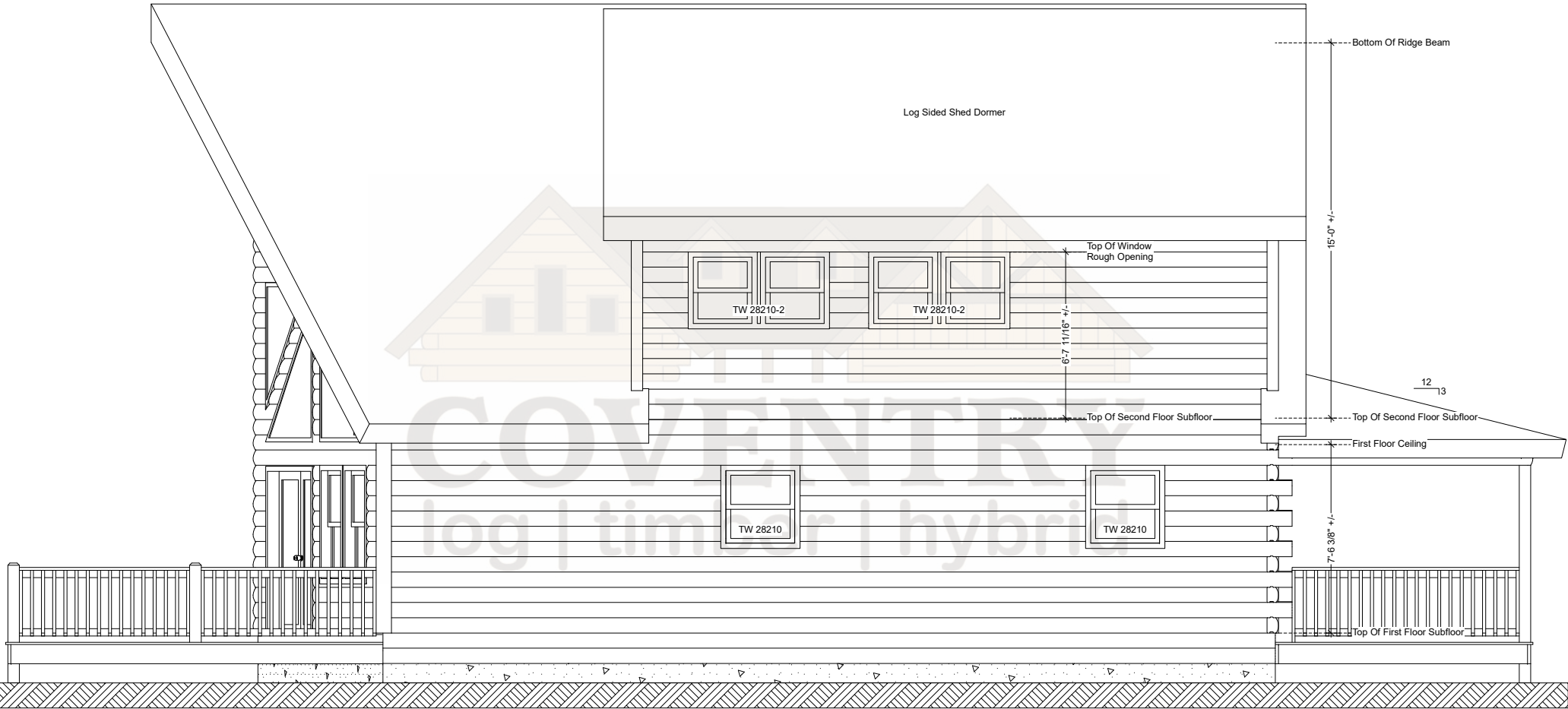
Aspen Right Elevation
