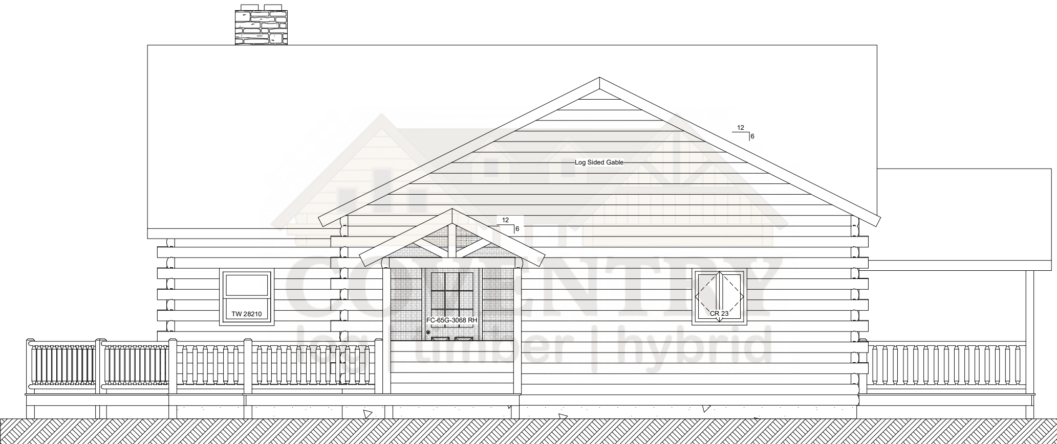
Big Sky Right Elevation
