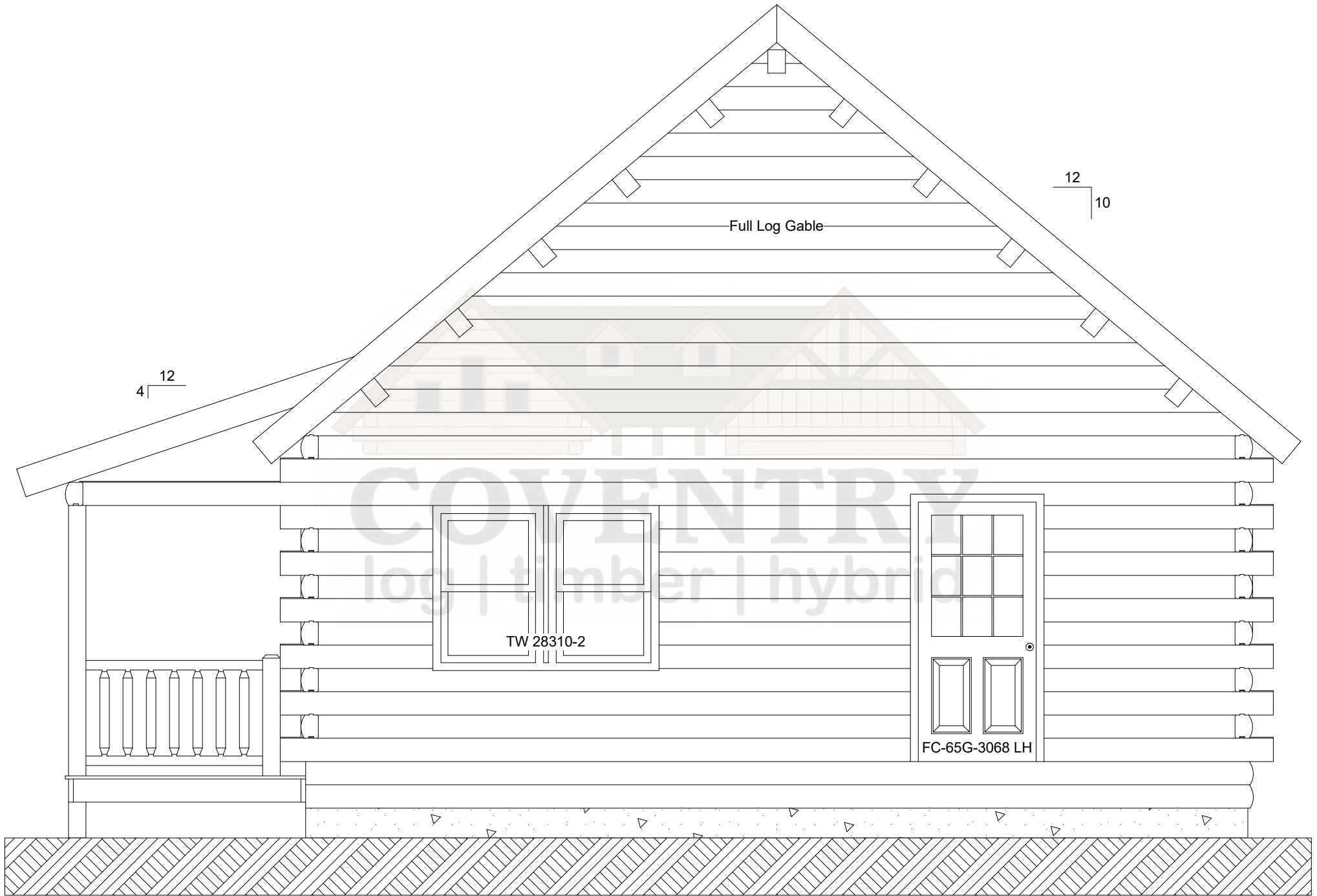
Hickory Right Elevation
