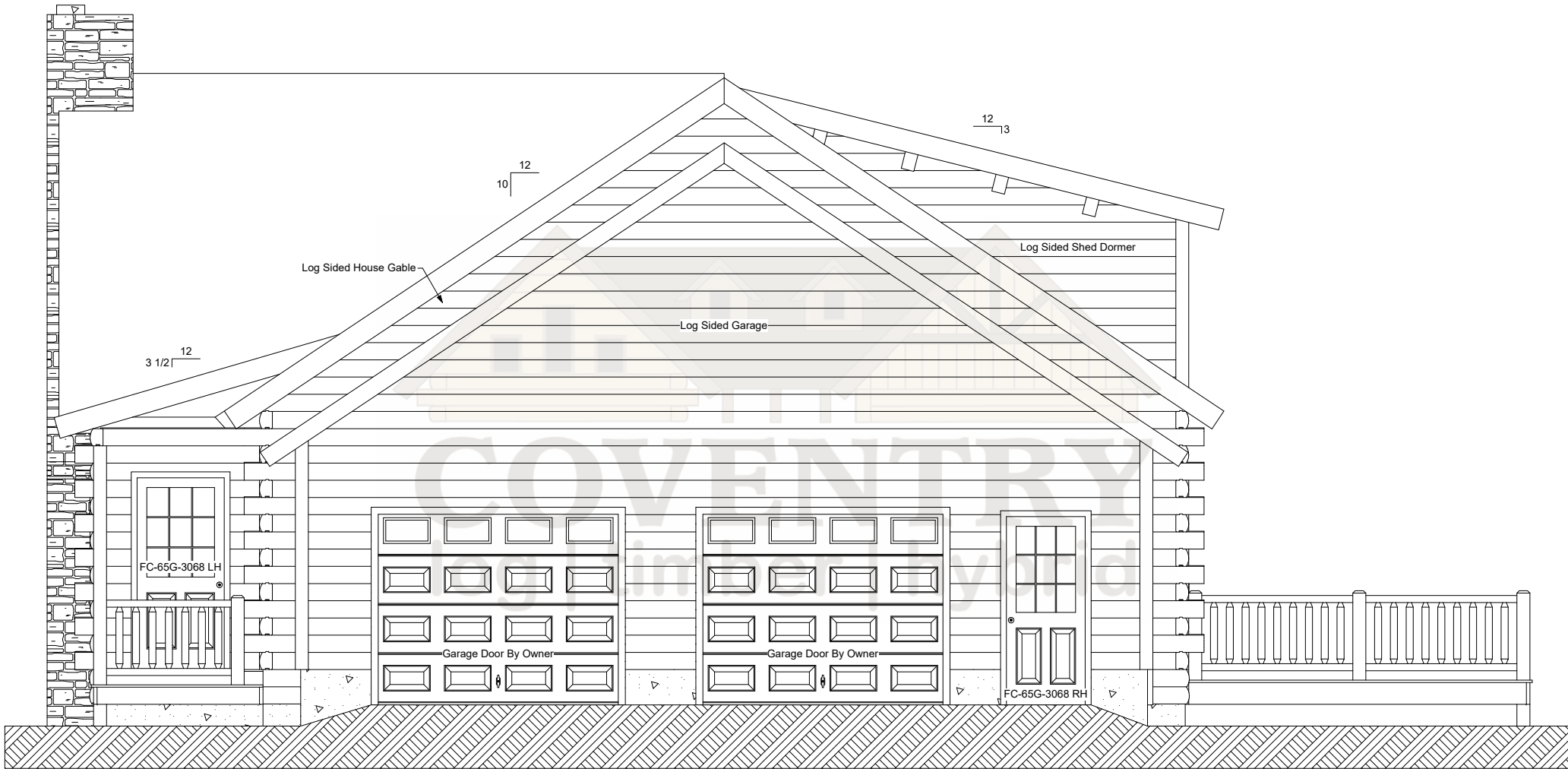
Sunapee Right Elevation
