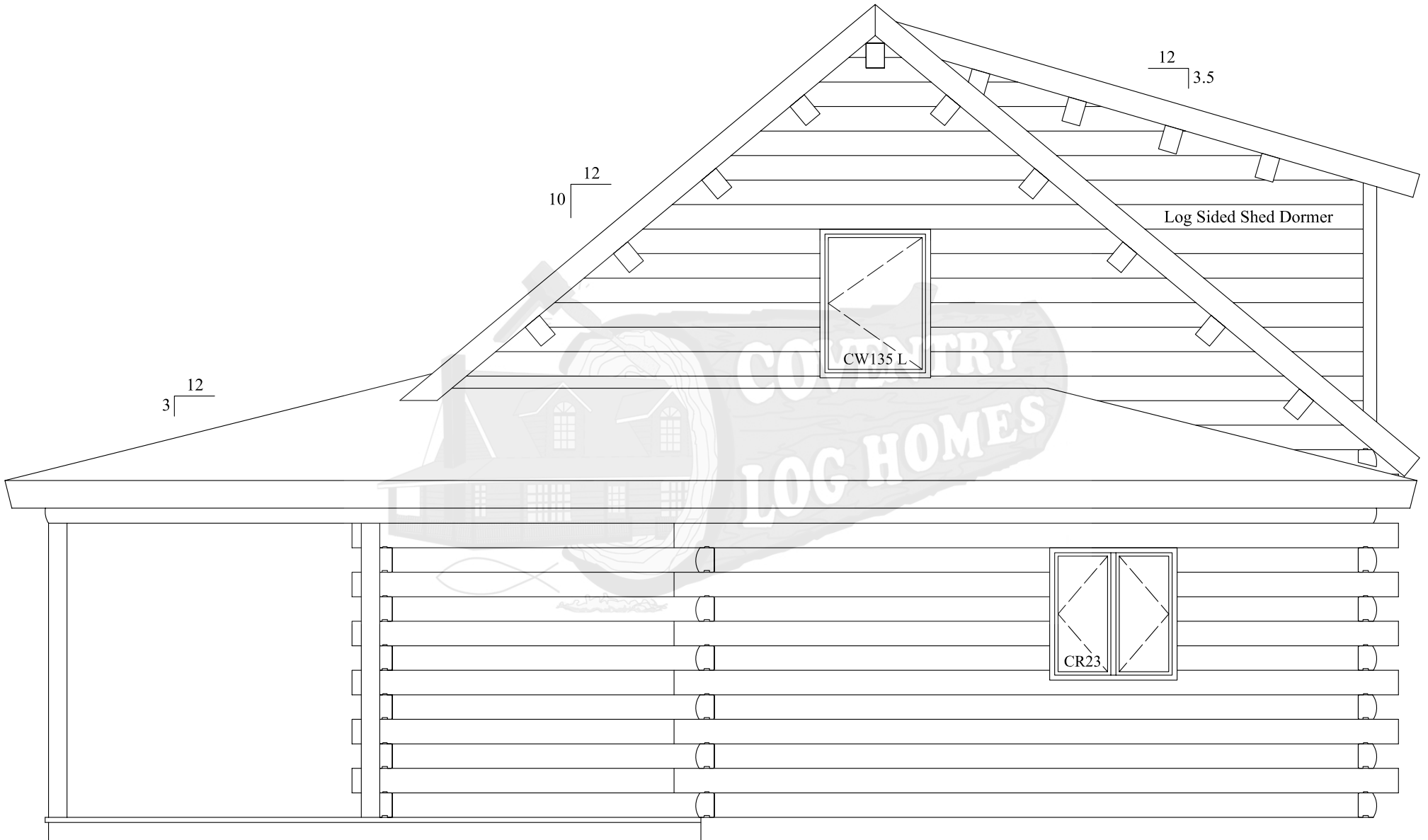
Right Elevation
