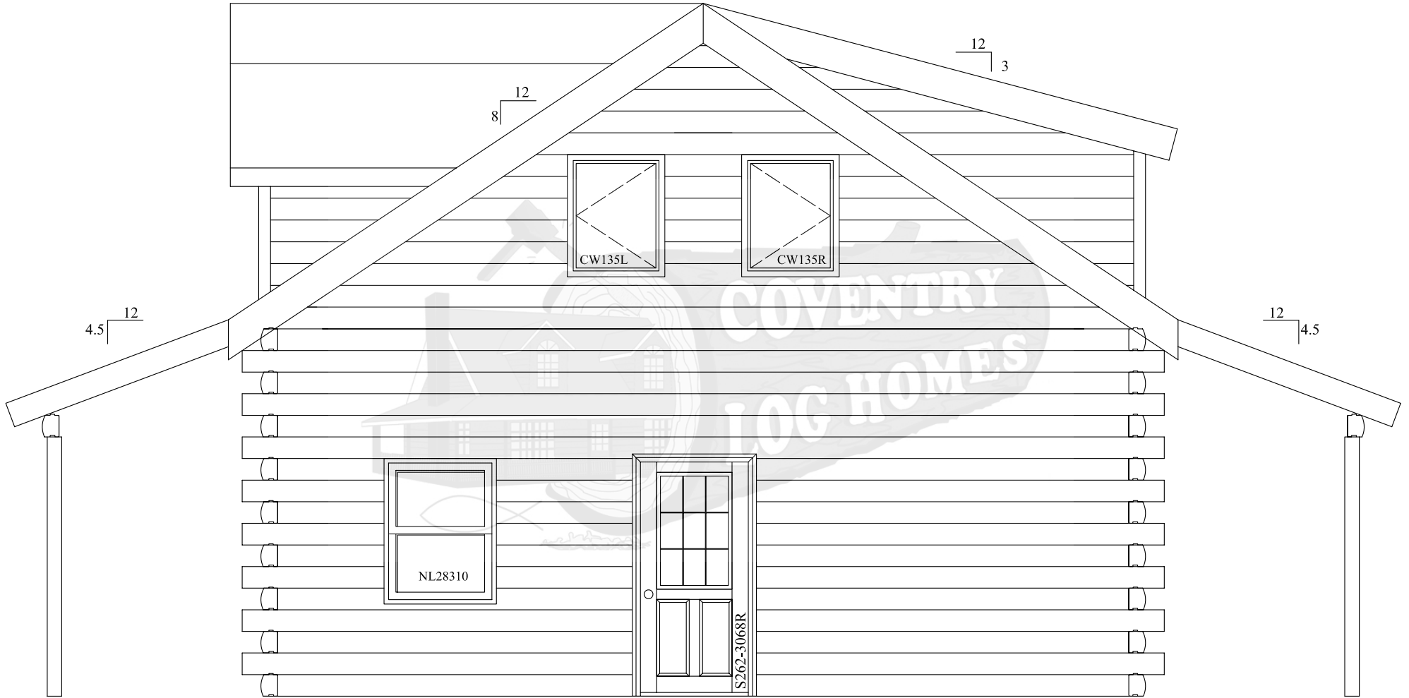
Elevation B
