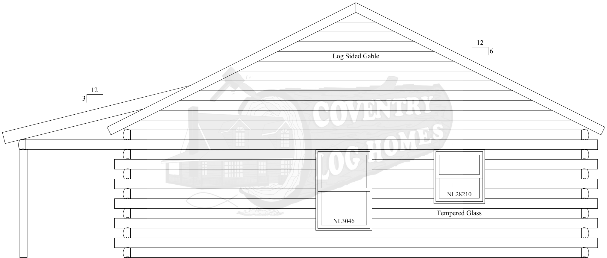
ELEVATION B
