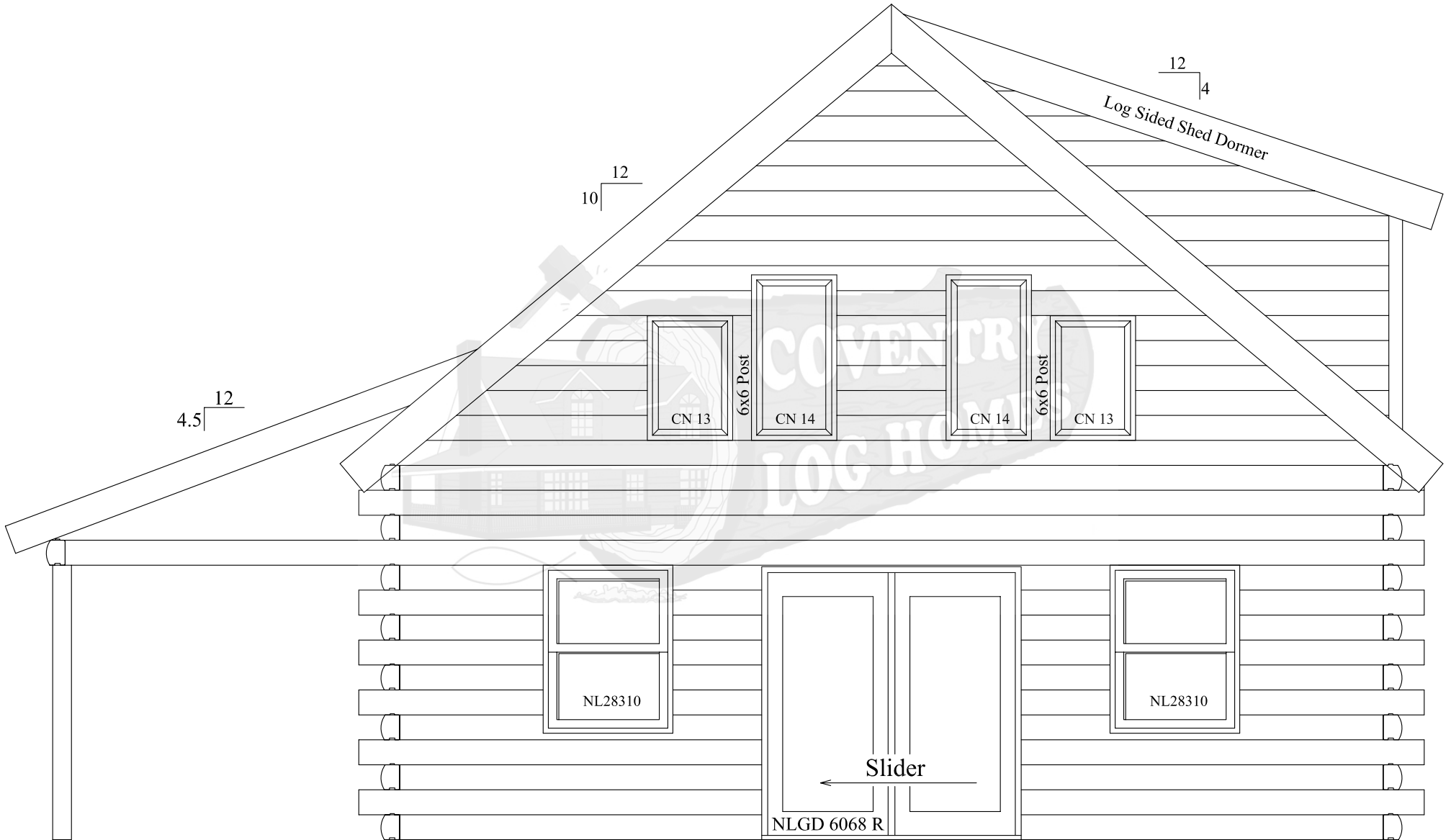
Elevation A
