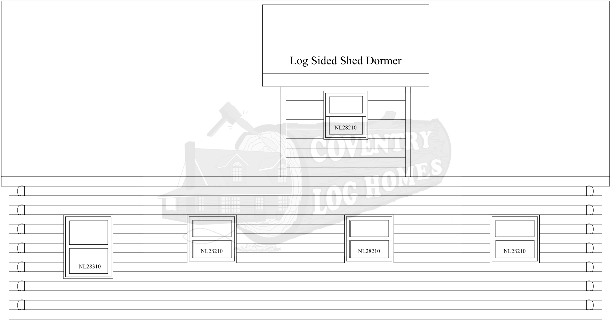
Elevation B
