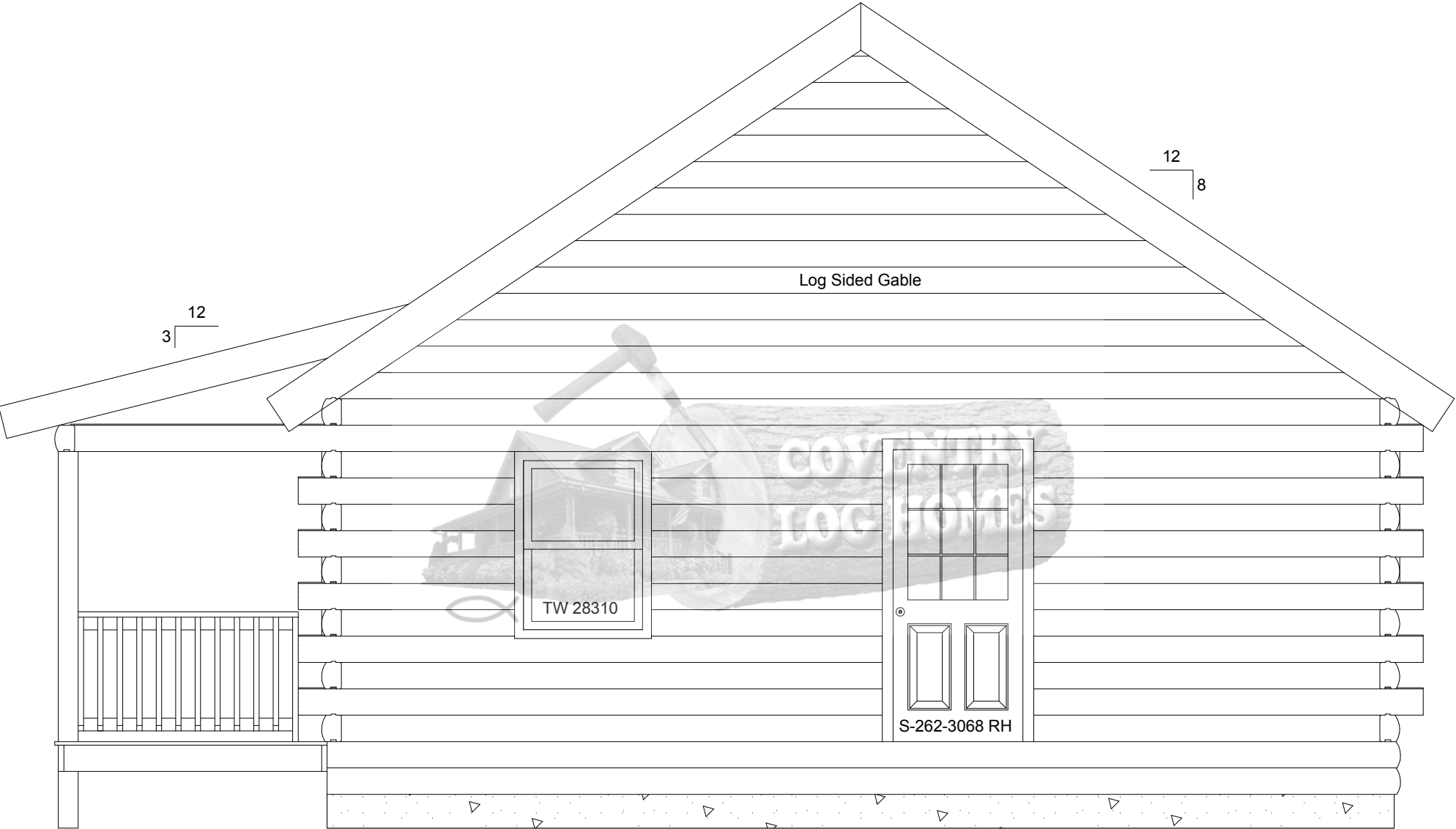
Right Elevation
